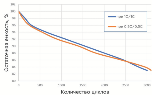
Количество циклов при 25°C и глубине разряда 100%
